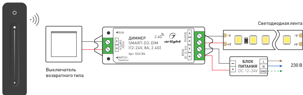
Рисунок 1. Схема подключения панели SMART-DIM-SET-LINE
