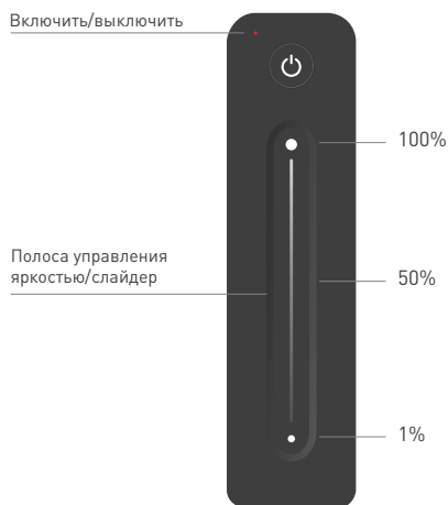
Рисунок 2. Назначение кнопок на пульте управления
