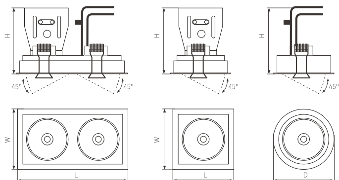
Рис. 1. Чертеж и габаритные размеры
