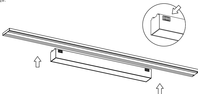
Рис. 2. Установка светильника
